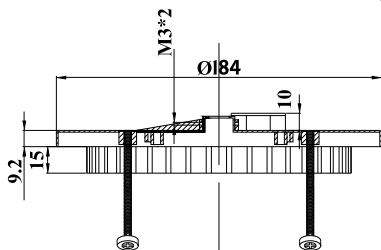
ODMP1325 (25W)
