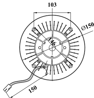
ODMP1325 (25W)
