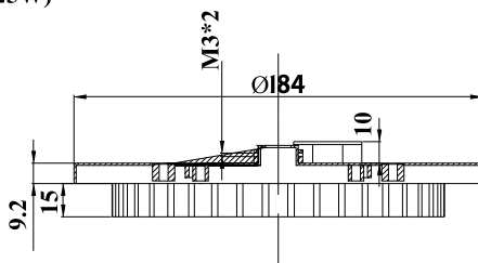
ODMP1325 (25W)
