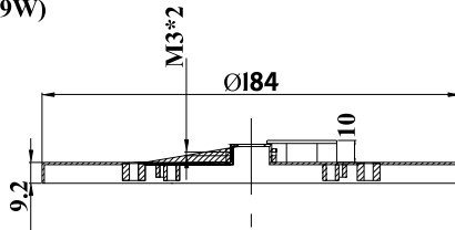
ODMP1319 (19W)
